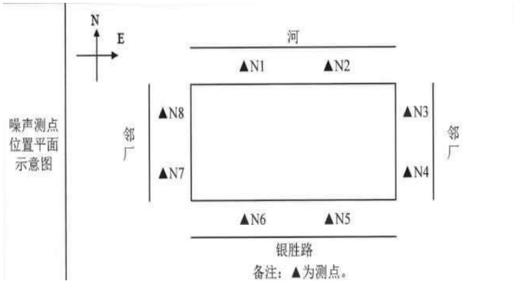
噪声污染检测点示意图
